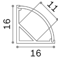
Aluprofil Weiß
